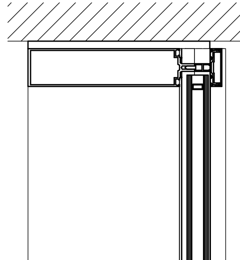
5 Detail 3 1 : 5
