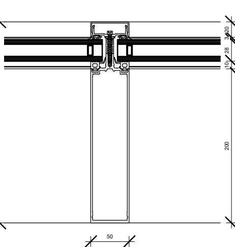
4 Detail 2 1 : 5
