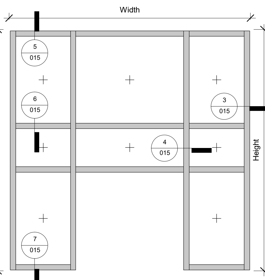
2 Elevation Back 1 : 20
