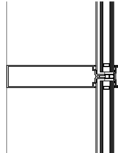
6 Detail 4 1 : 5
