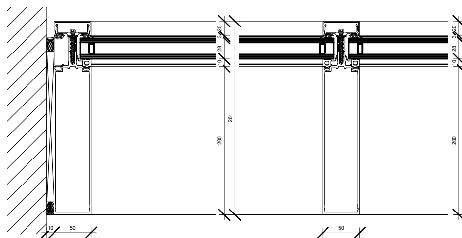
3 Detail 1 1 : 5
